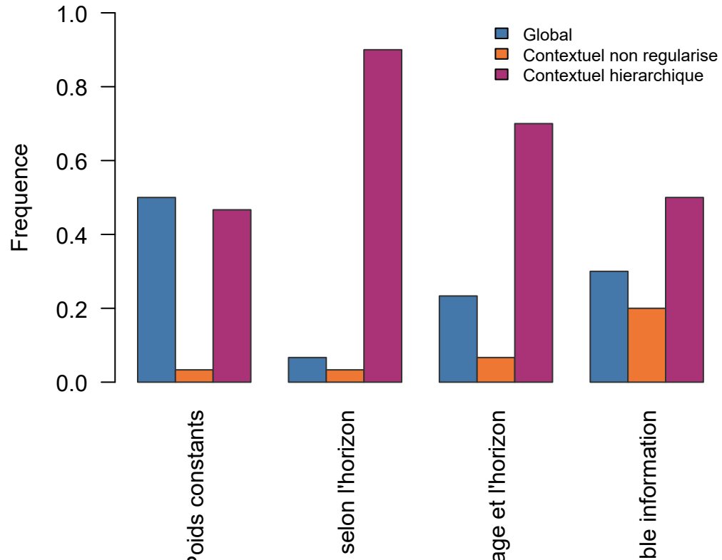
Meilleur CRPS
