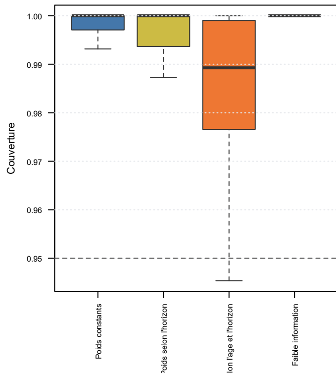
Couverture des intervalles a 95 %
