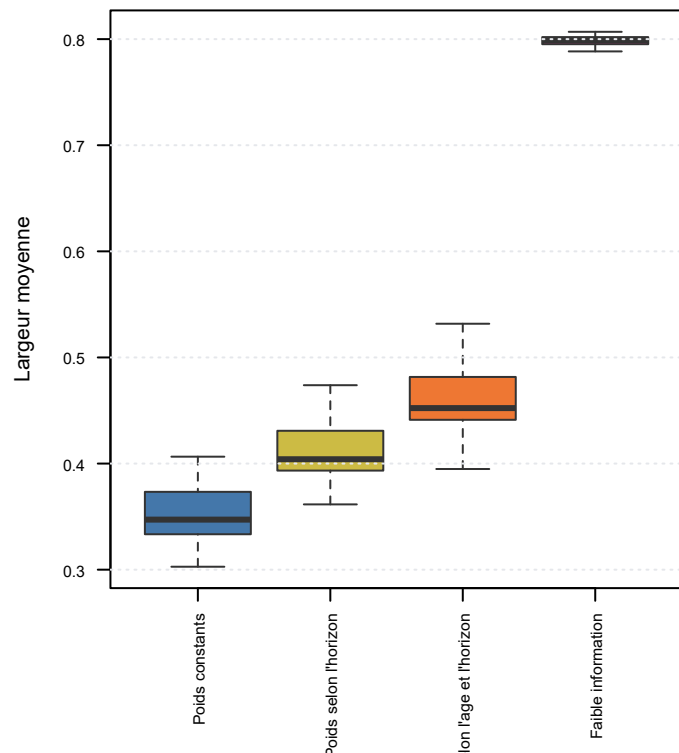
Largeur des intervalles credibles
