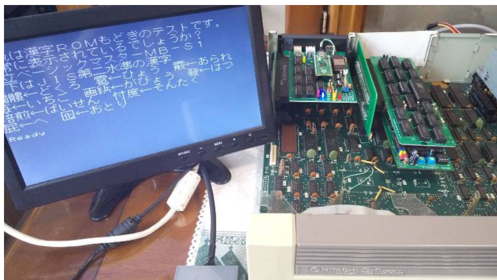
図 2: S1 本体で動作確認
