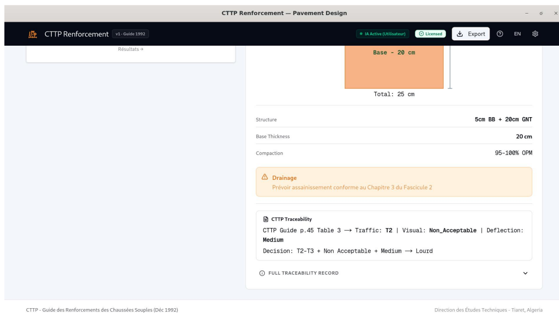
Figure 1.14. Structure de renforcement candidate : type Lourd , GNT, coupe transversale 5 cm BB + 20 cm GNT, compactage 95-100 % OPM et alerte de drainage.
