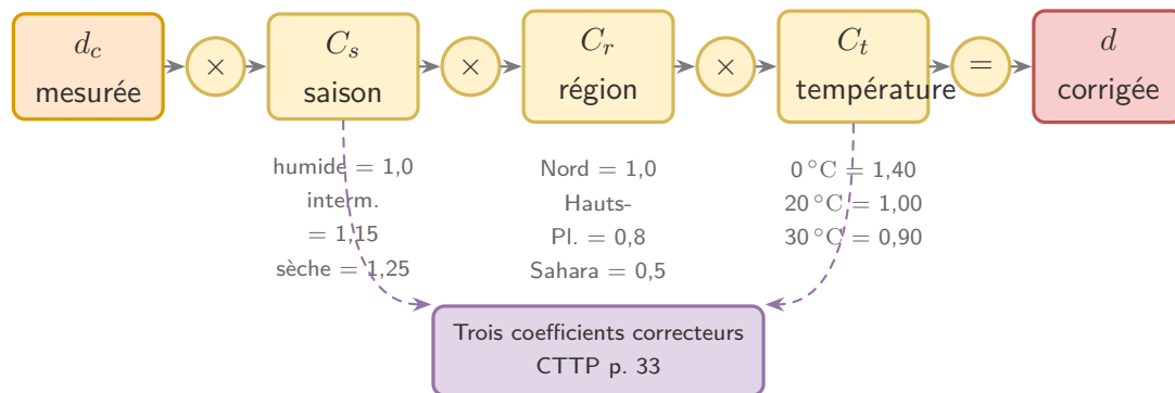
Figure 1.4. Schéma de calcul de la déflexion corrigée (diagramme Mermaid) : d = d_c \times C_s \times C_r \times C_t (d'après CTTTP p. 33).
