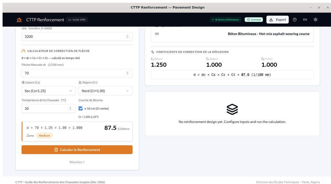
Figure 1.12. Calculateur de correction de flèche : affichage explicite de d_c , C_s , C_r , C_t et de la déflexion corrigée d = 70 \times 1,25 \times 1,00 \times 1,000 = 87,5 (zone Medium).
