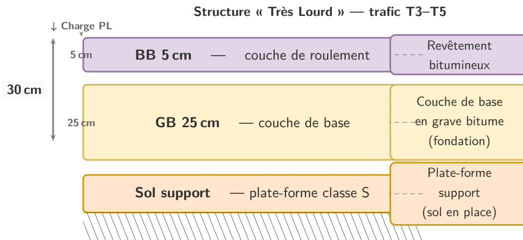
Figure 1.5. Coupe transversale type d’une structure de renforcement « Très Lourd » pour un trafic T3–T5 (d’après CTTP p. 48–55, diagramme Mermaid).
