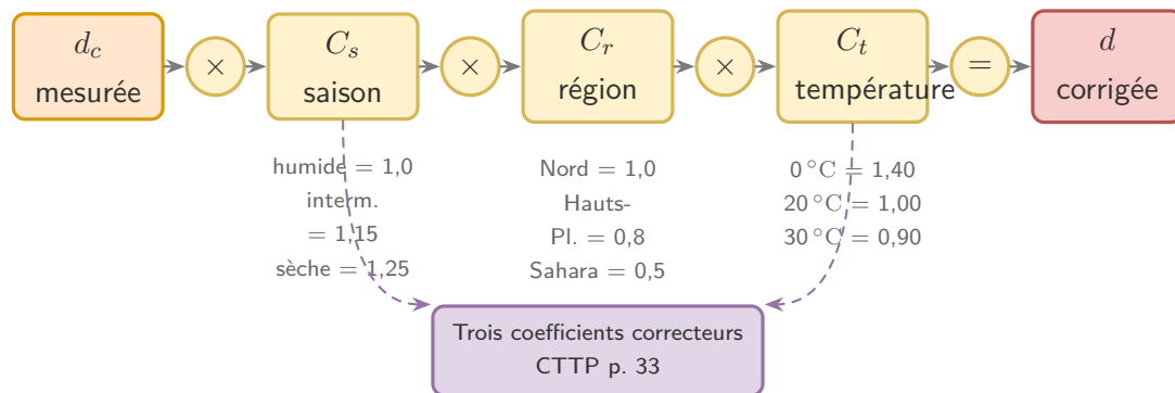
Figure 1.4. Schéma de calcul de la déflexion corrigée (diagramme Mermaid) : d = d_c \times C_s \times C_r \times C_t (d'après CTTP p. 33).
