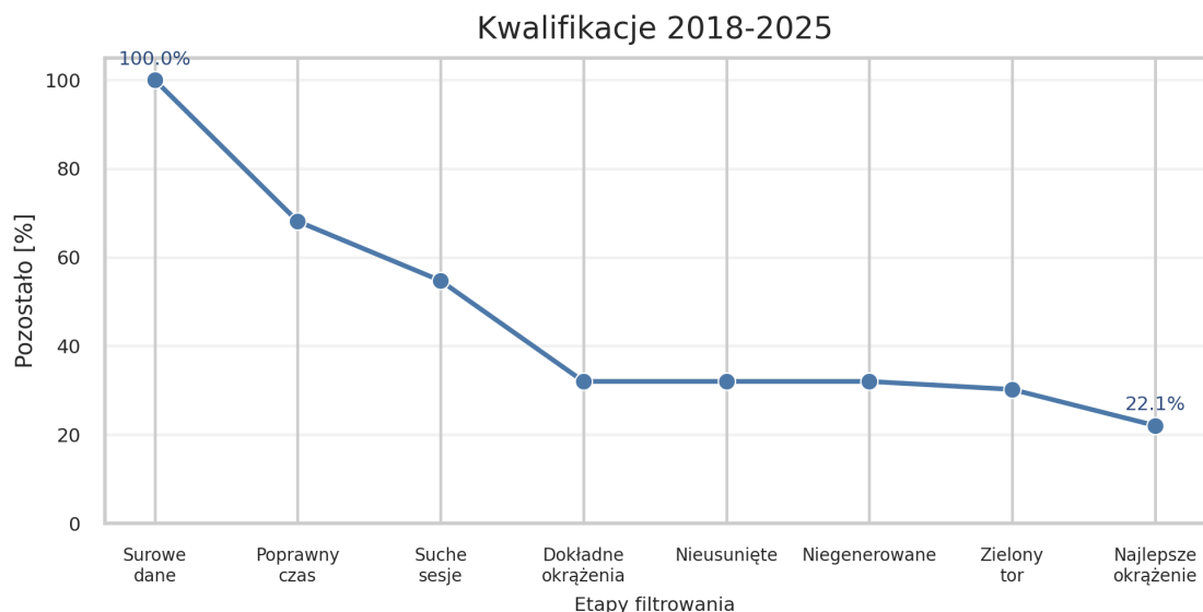
Rysunek 3.3 Redukcja danych po kolejnych filtrach w setupie kwalifikacyjnym 2018–2025.
