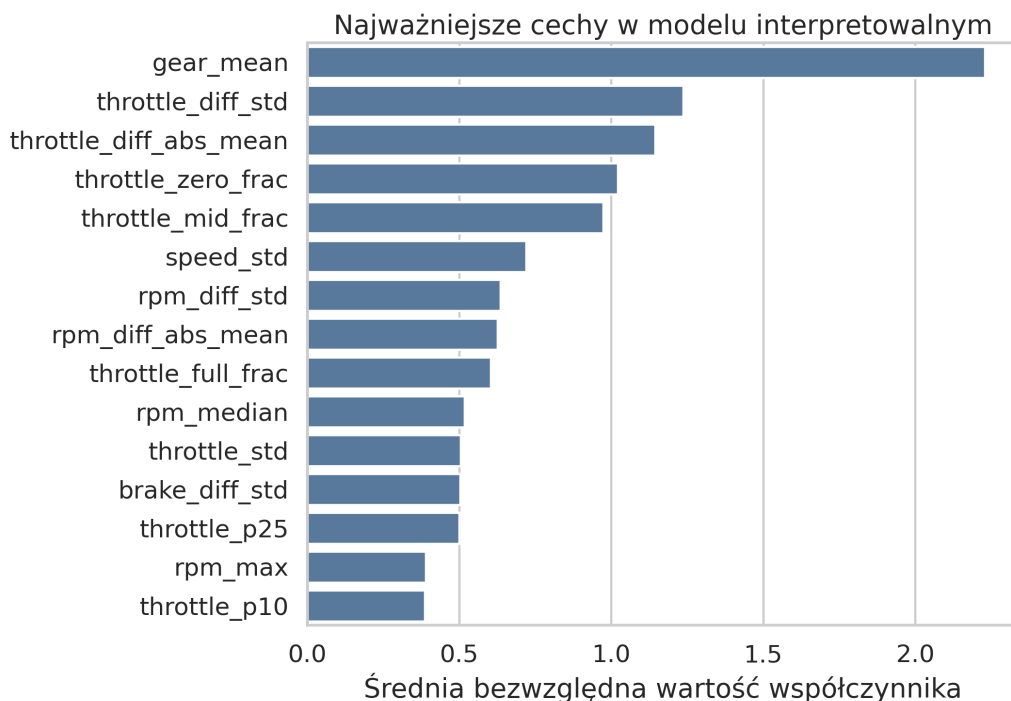
Rysunek 5.8 Najważniejsze cechy w modelu interpretowalnym.
