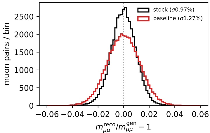
A. ATLAS muon revision (Z, barrel)
