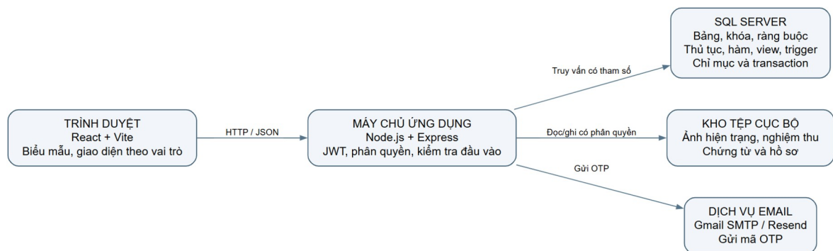
Hình 5.1. Kiến trúc ứng dụng HomeFix
