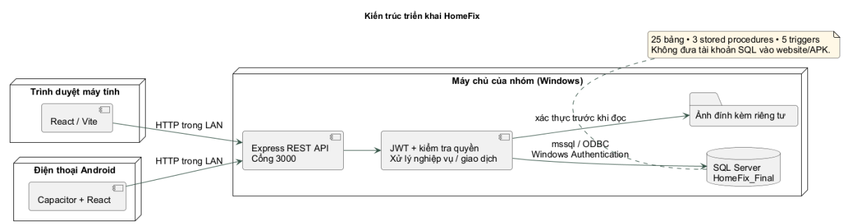
Hình 5.1. Kiến trúc triển khai
