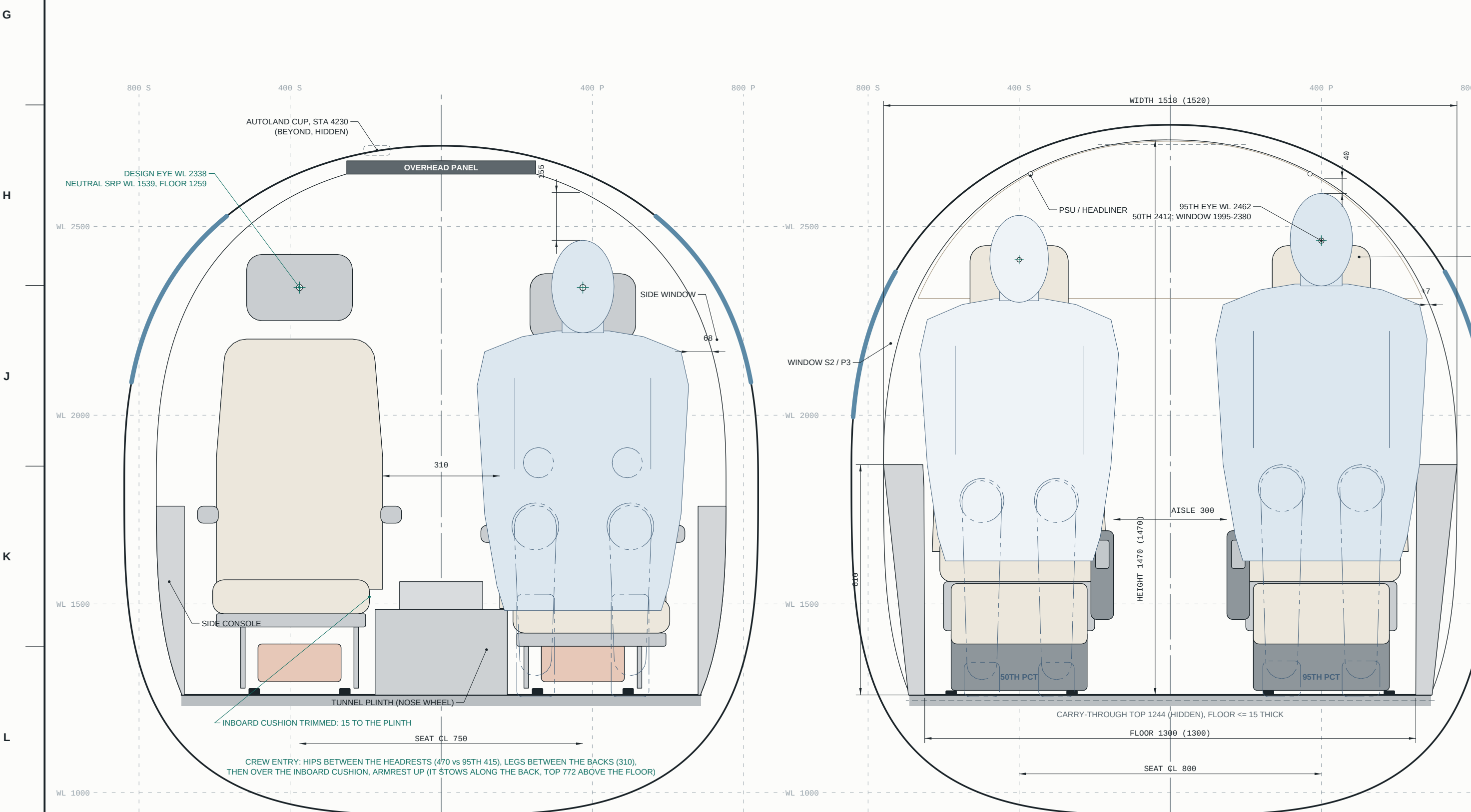
SECTION A-A
