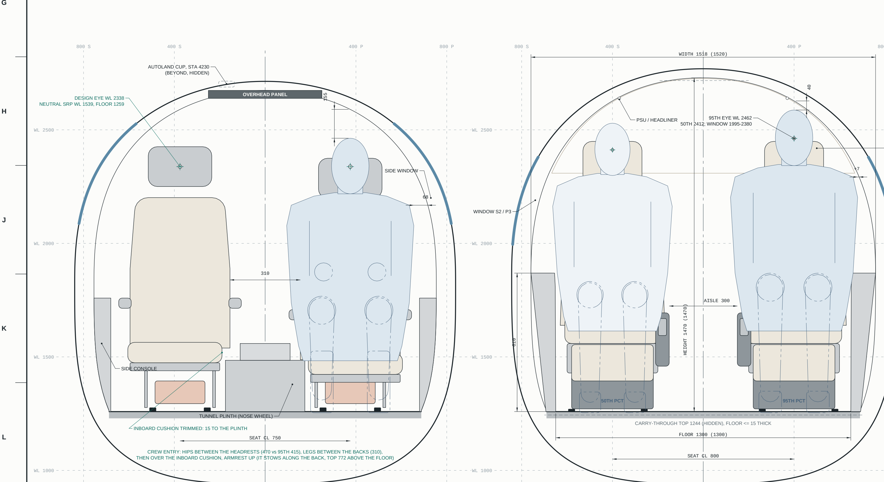
SECTION A-A
