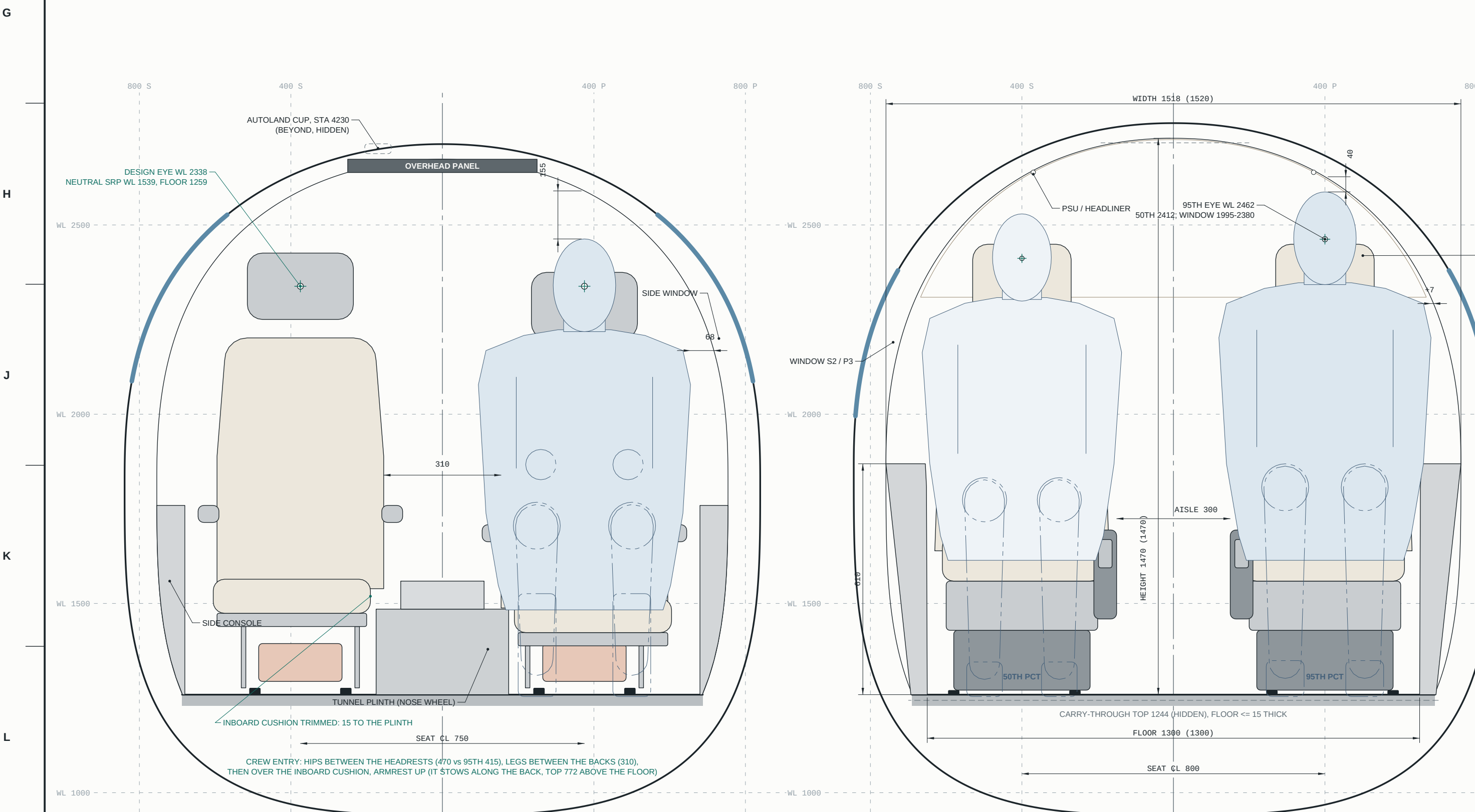
SECTION A-A
