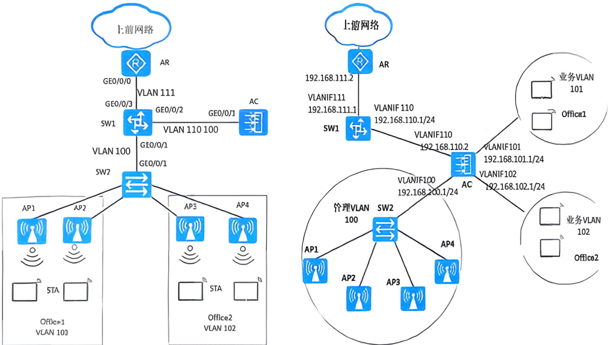
图 2 网络拓扑
