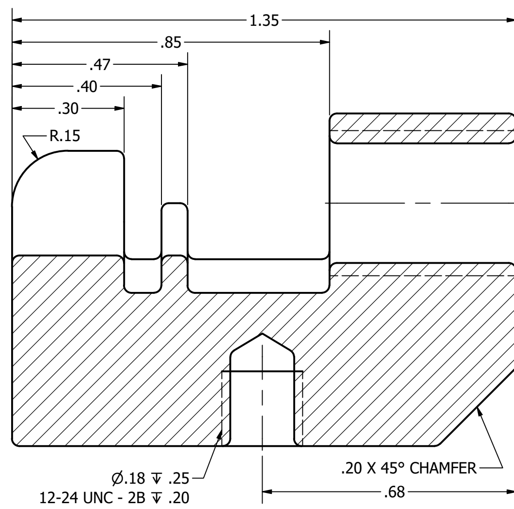
SECTION A-A
