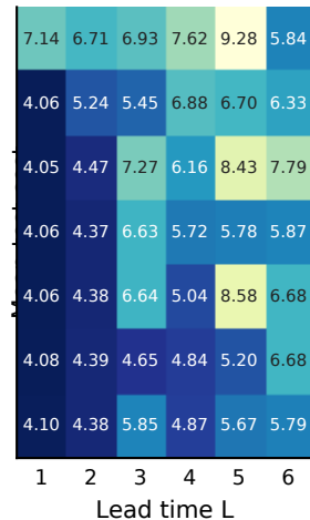
No DCA
