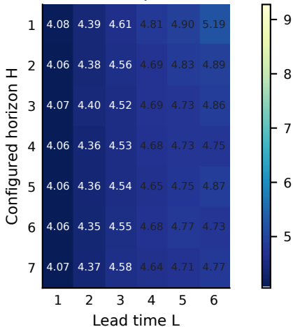
MDQN
