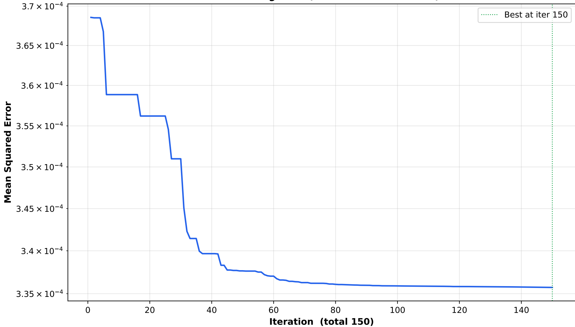
PSO Convergence (best MSE = 3.357e-04)
