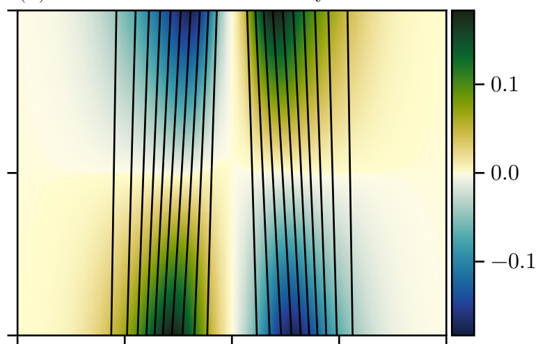
(d) Filament vertical viscosity
