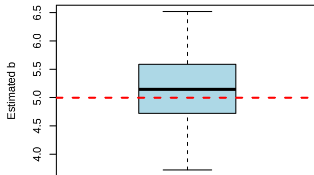
Scenario 2: b (True = 5)
