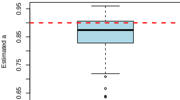
Scenario 1: a (True = 0.9)
