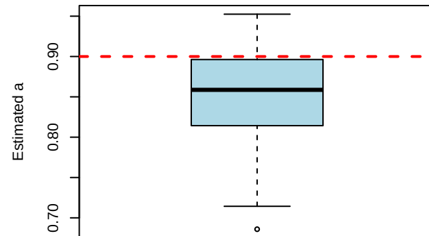
Scenario 3: a (True = 0.9)
