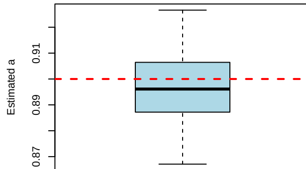
Scenario 2: a (True = 0.9)
