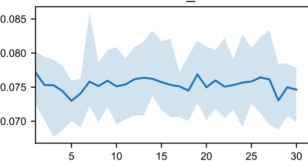
test_pred_time
