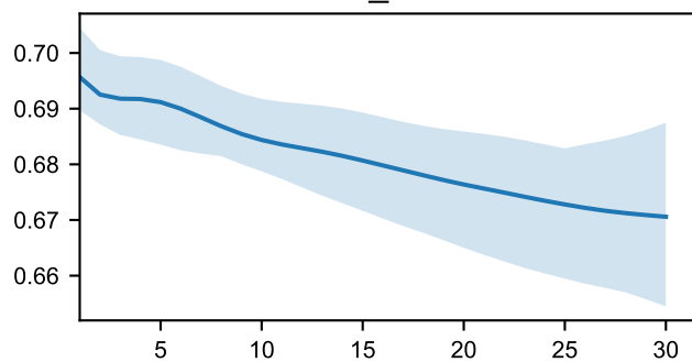
val_auc
