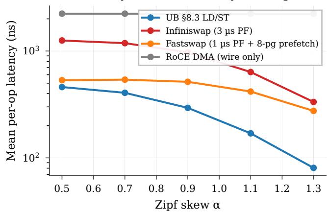
(d) Latency vs skew (64 K-key working set)
