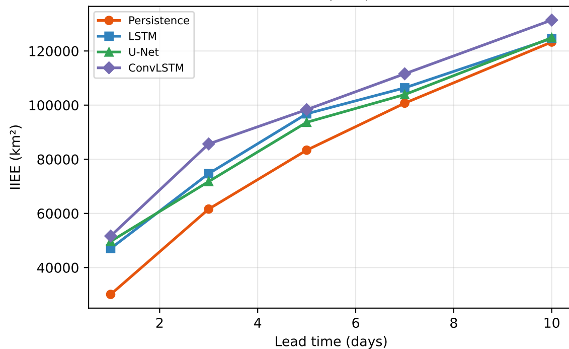
IIEE (km 2 )
