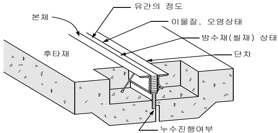
< 신축이음 점검부위 >
