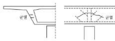
< 정착구역의 국부균열 >
