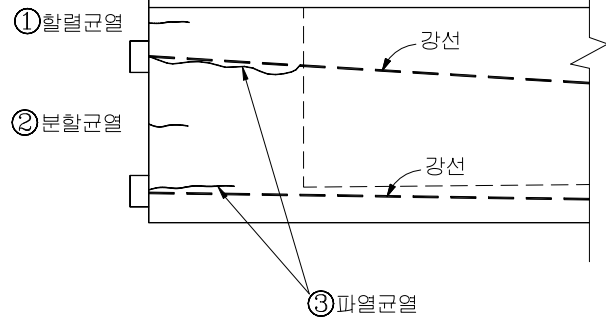
< 정착구역의 국부균열 >
