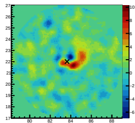
ResidualSig 100&lt;=nhit&lt;200
