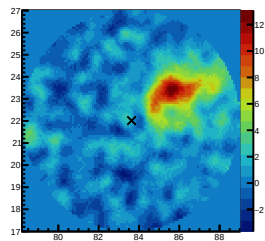
ResidualSig 25.12TeV&lt;E&lt;39.81TeV
