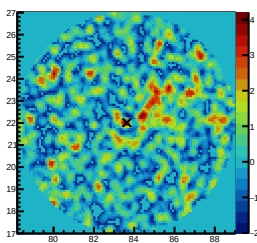
ResidualSig 100.00TeV&lt;E&lt;158.49TeV
