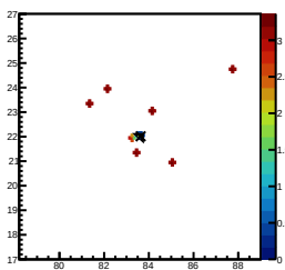
ResidualSig 1000.00TeV&lt;E&lt;1584.89TeV
