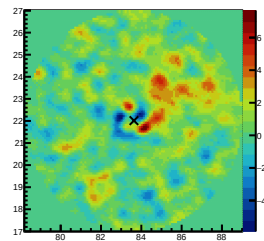
ResidualSig 200&lt;=nhit&lt;300
