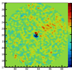
ResidualSig 800&lt;=nhit&lt;2000
