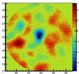
ResidualSig 30&lt;=nhit&lt;60
