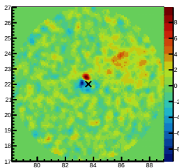
ResidualSig 500&lt;=nhit&lt;800
