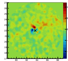
ResidualSig 300&lt;=nhit&lt;500
