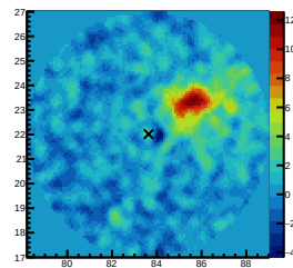
ResidualSig 39.81TeV&lt;E&lt;63.10TeV
