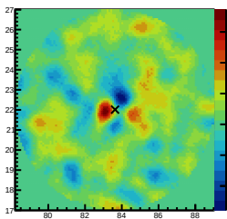
ResidualSig 60&lt;=nhit&lt;100
