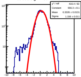
ResidualSig1D 30&lt;=nhit&lt;60
