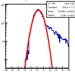
ResidualSig1D 25.12TeV&lt;E&lt;39.81TeV
