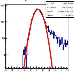
ResidualSig1D 39.81TeV&lt;E&lt;63.01TeV
