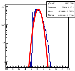
ResidualSig1D 100.00TeV&lt;E&lt;158.49TeV
