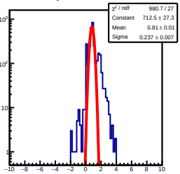
ResidualSig1D 158.49TeV&lt;E&lt;251.19TeV
