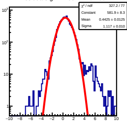
ResidualSig1D 100&lt;=nhit&lt;200
