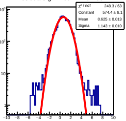
ResidualSig1D 60&lt;=nhit&lt;200
