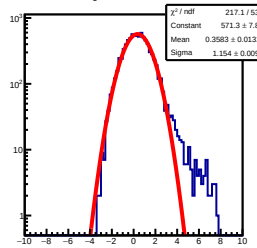
ResidualSig1D 63.01TeV&lt;E&lt;100.00TeV
