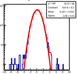
ResidualSig1D 800&lt;=nhit&lt;2000
