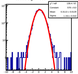
ResidualSig1D 500&lt;=nhit&lt;800
