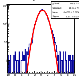
ResidualSig1D 300&lt;=nhit&lt;500
