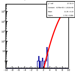
ResidualSig1D 1000.00TeV&lt;E&lt;1584.89TeV
