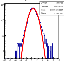
ResidualSig1D 200&lt;=nhit&lt;300
