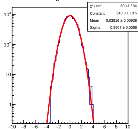
ResidualSig1D 200&lt;=nhit&lt;300
