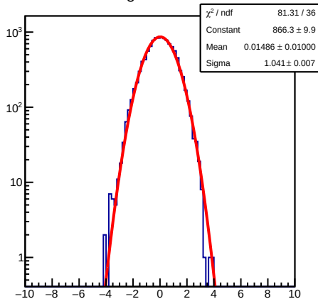
ResidualSig1D 500&lt;=nhit&lt;800
