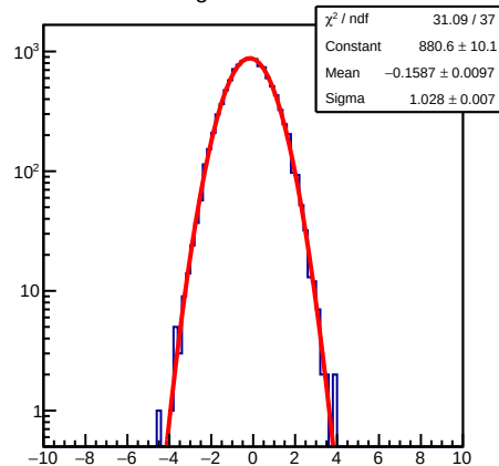
ResidualSig1D 800&lt;=nhit&lt;2000
