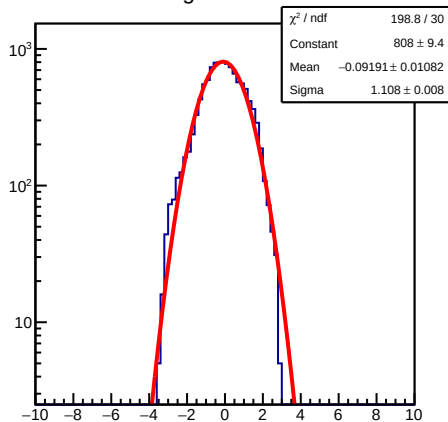
ResidualSig1D 60&lt;=nhit&lt;100
