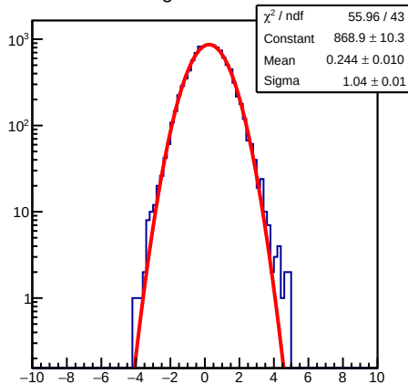
ResidualSig1D 300&lt;=nhit&lt;500
