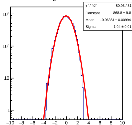
ResidualSig1D 100&lt;=nhit&lt;200
