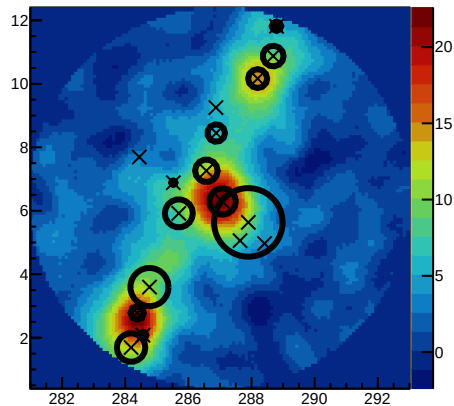
DataSig 60&lt;=nhit&lt;100
