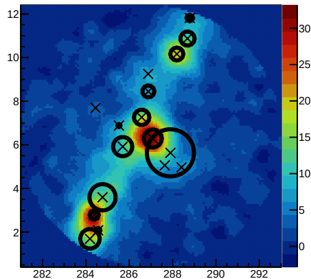
DataSig 100&lt;=nhit&lt;200
