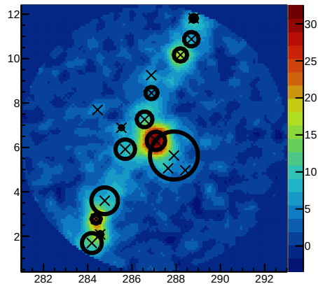
DataSig 300&lt;=nhit&lt;500
