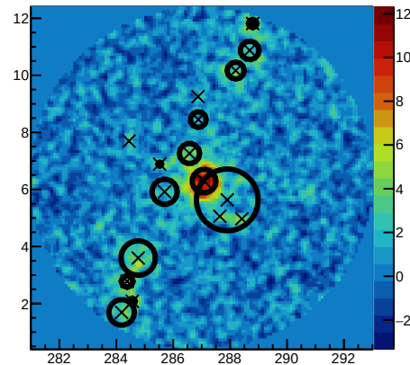
DataSig 800&lt;=nhit&lt;2000
