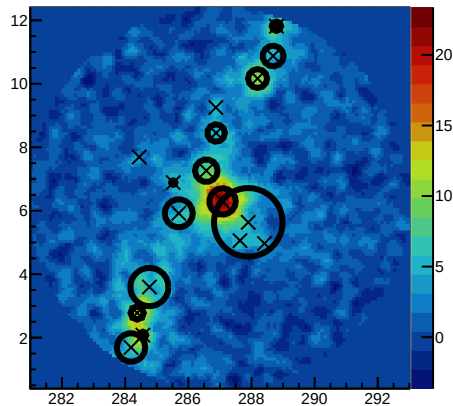
DataSig 500&lt;=nhit&lt;800
