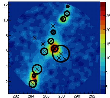
DataSig 200&lt;=nhit&lt;300
