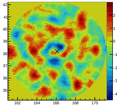
ResidualSig 100&lt;=nhit&lt;200
