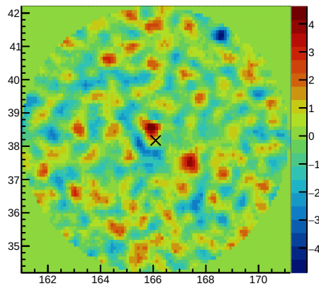
ResidualSig 500&lt;=nhit&lt;800
