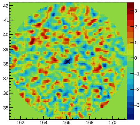
ResidualSig 800&lt;=nhit&lt;2000
