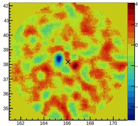
ResidualSig 200&lt;=nhit&lt;300
