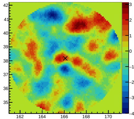
ResidualSig 60&lt;=nhit&lt;100
