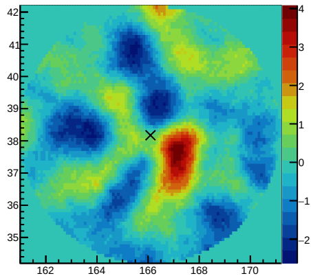
ResidualSig 30&lt;=nhit&lt;60
