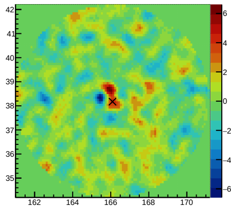
ResidualSig 300&lt;=nhit&lt;500
