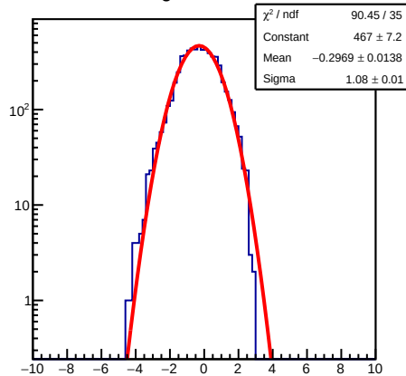
ResidualSig1D 100&lt;=nhit&lt;200
