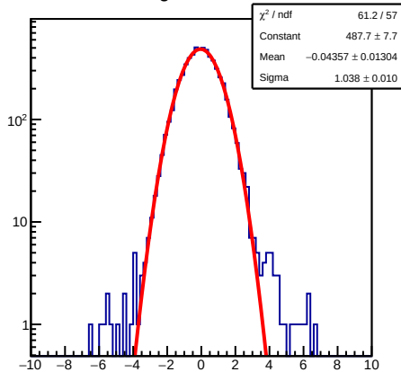
ResidualSig1D 300&lt;=nhit&lt;500
