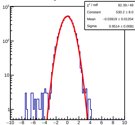
ResidualSig1D 200&lt;=nhit&lt;300
