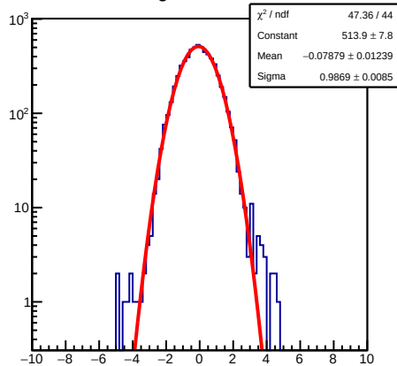
ResidualSig1D 500&lt;=nhit&lt;800
