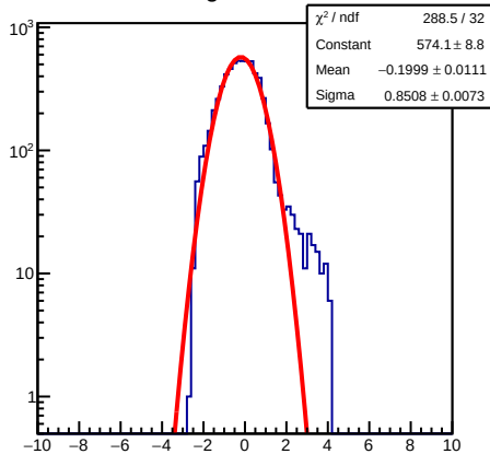
ResidualSig1D 30&lt;=nhit&lt;60
