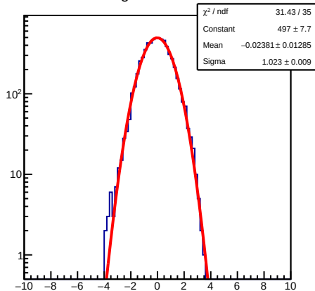
ResidualSig1D 800&lt;=nhit&lt;2000
