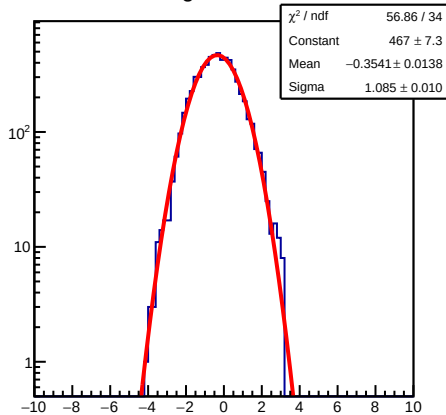
ResidualSig1D 60&lt;=nhit&lt;100
