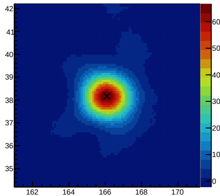
DataSig 30&lt;=nhit&lt;60
