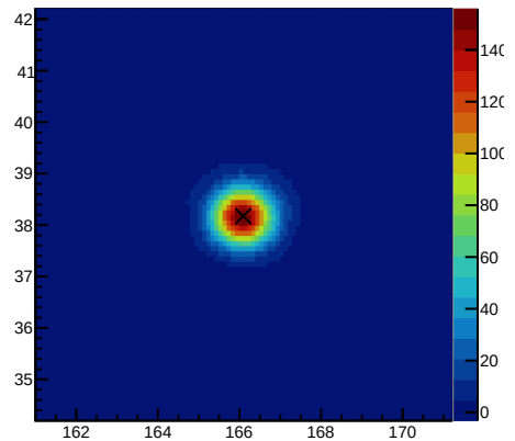
DataSig 100&lt;=nhit&lt;200
