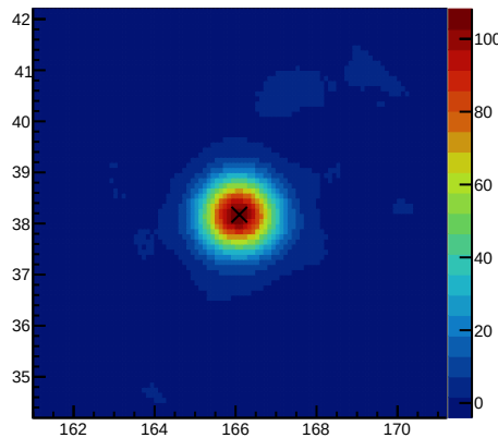
DataSig 60&lt;=nhit&lt;100
