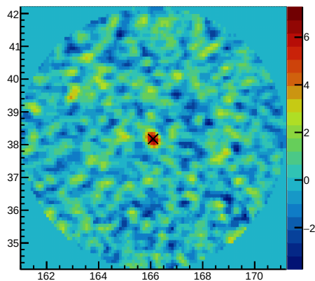
DataSig 800&lt;=nhit&lt;2000
