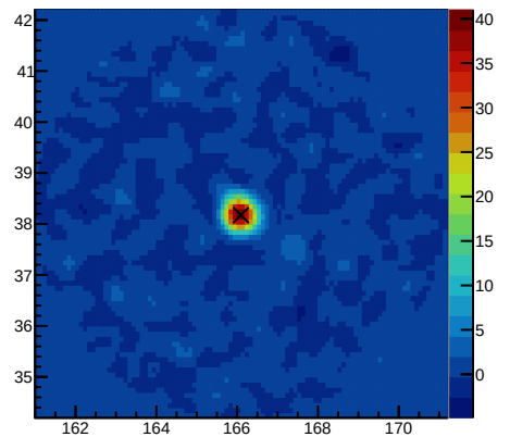
DataSig 500&lt;=nhit&lt;800
