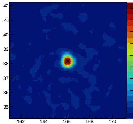
DataSig 300&lt;=nhit&lt;500
