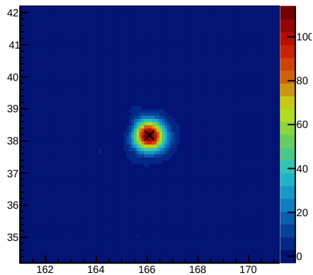
DataSig 200&lt;=nhit&lt;300
