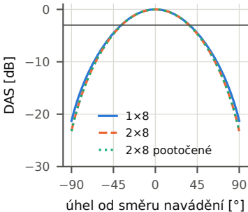
řez azimutem
