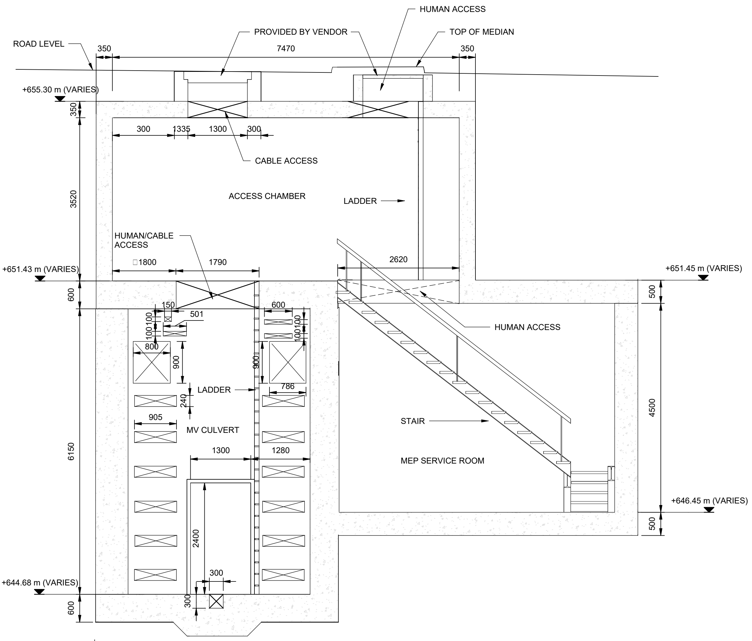
2 SECTION 1 : 50
