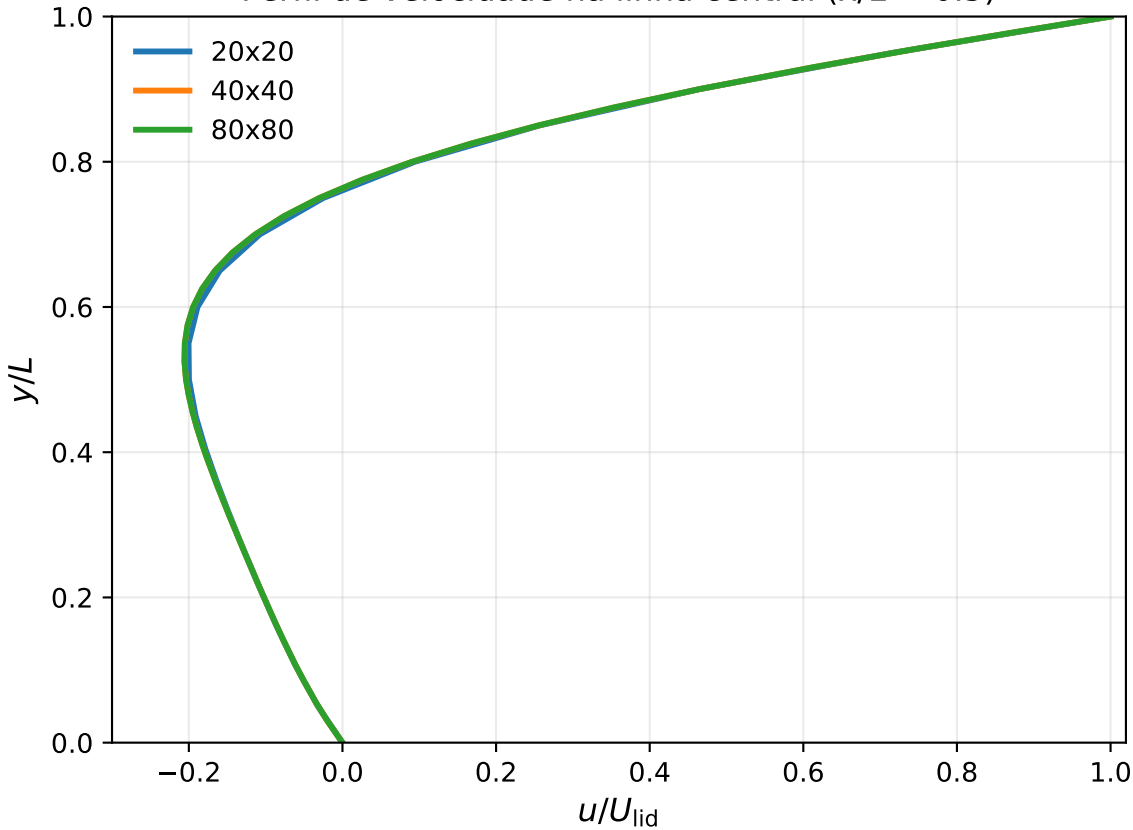
Perfil de velocidade na linha central ( x/L = 0.5 )
