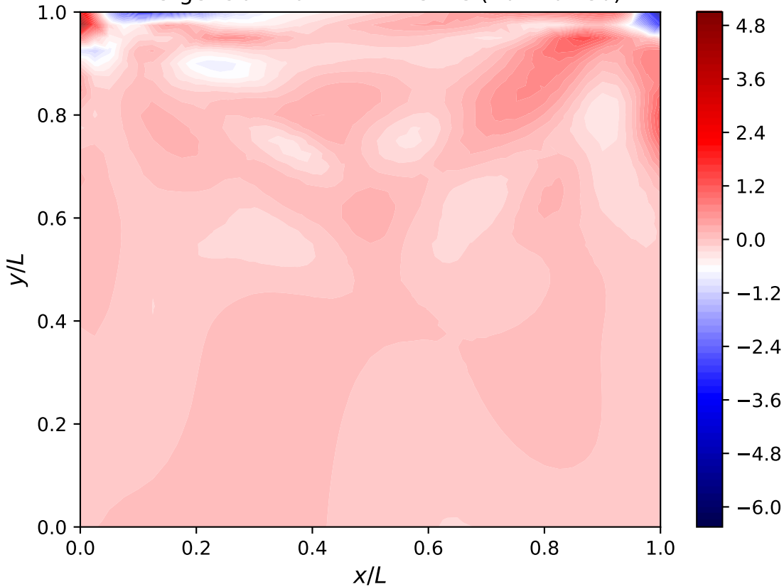
Divergência \nabla \cdot \mathbf{u} — MLP Refine (20→40→80)
