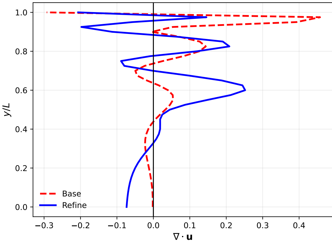
Perfil de divergência no centerline ( x/L = 0.5 )
