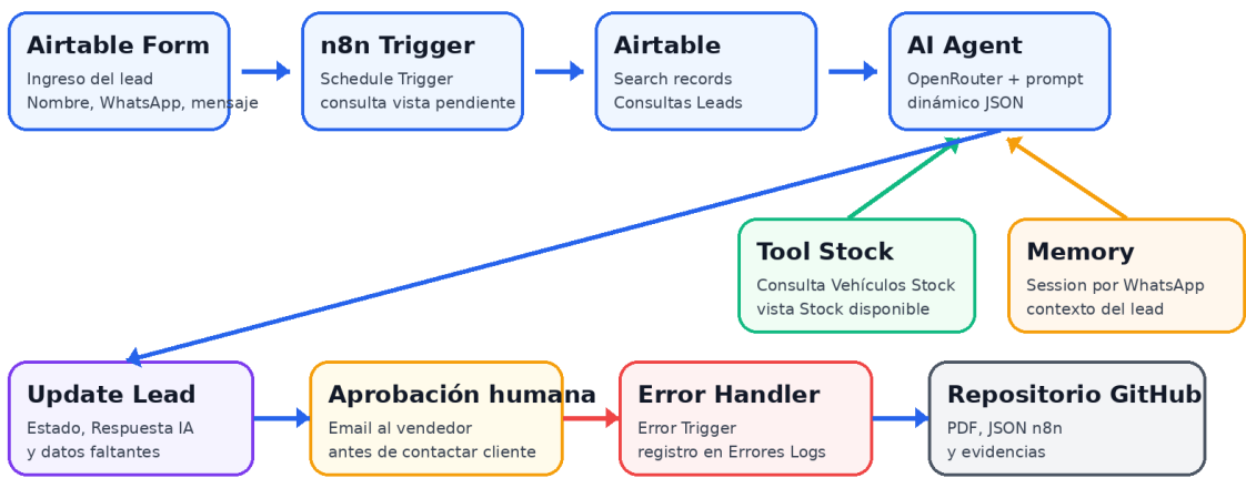
Figura 1. Arquitectura end-to-end del ecosistema de automatización IA.
