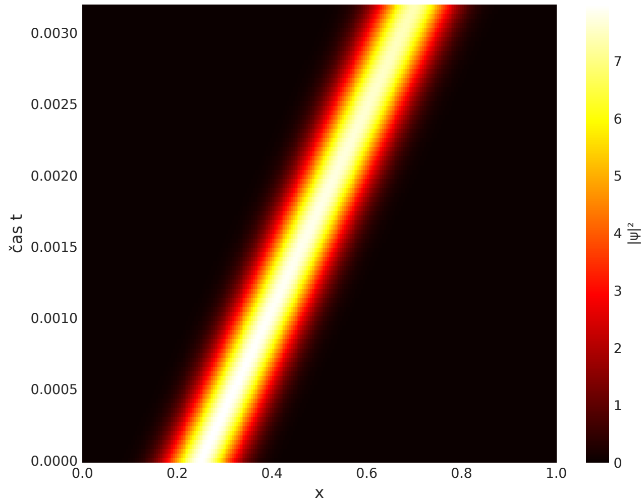
Absolutna vrednost valovne funkcije
