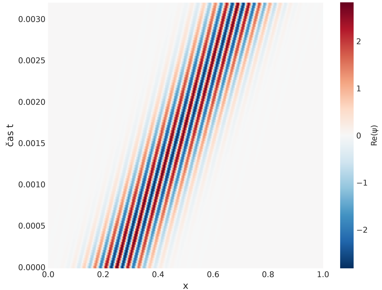
Realni del valovne funkcije
