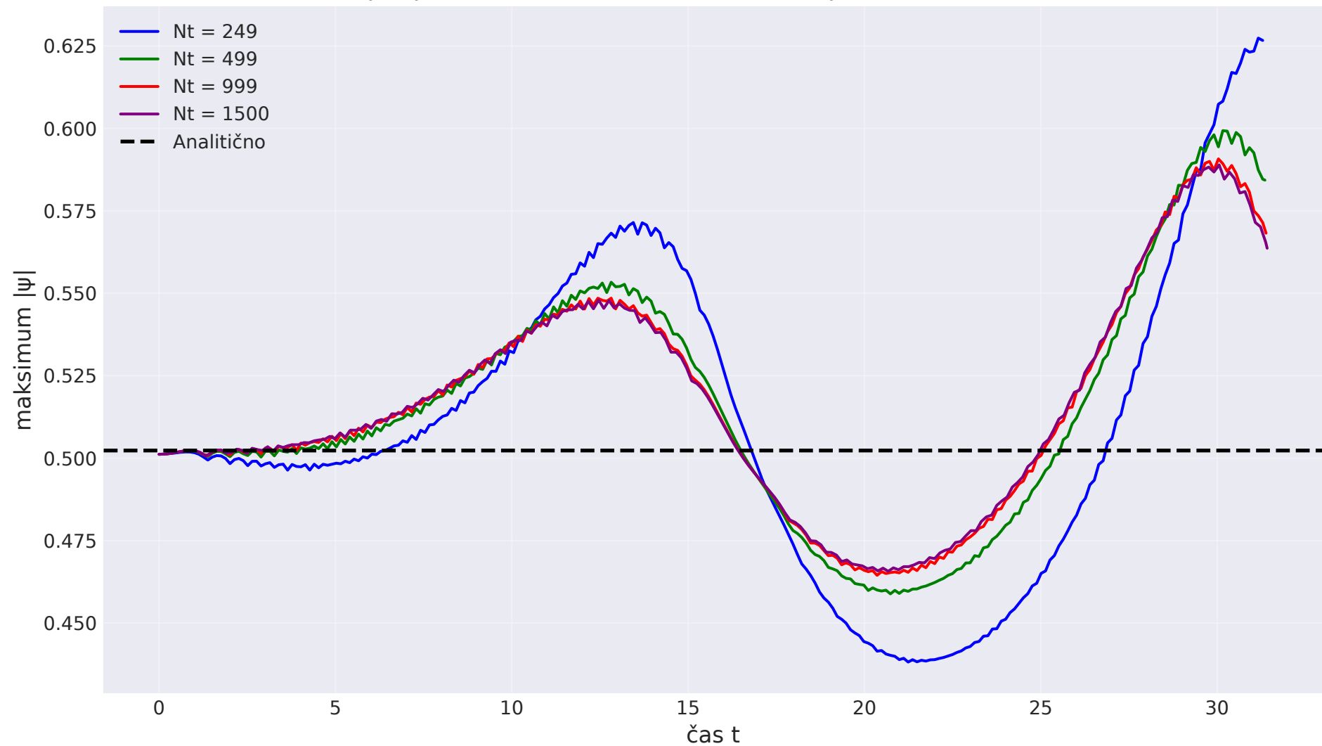
Največja absolutna vrednost valovne funkcije v odvisnosti od časa
