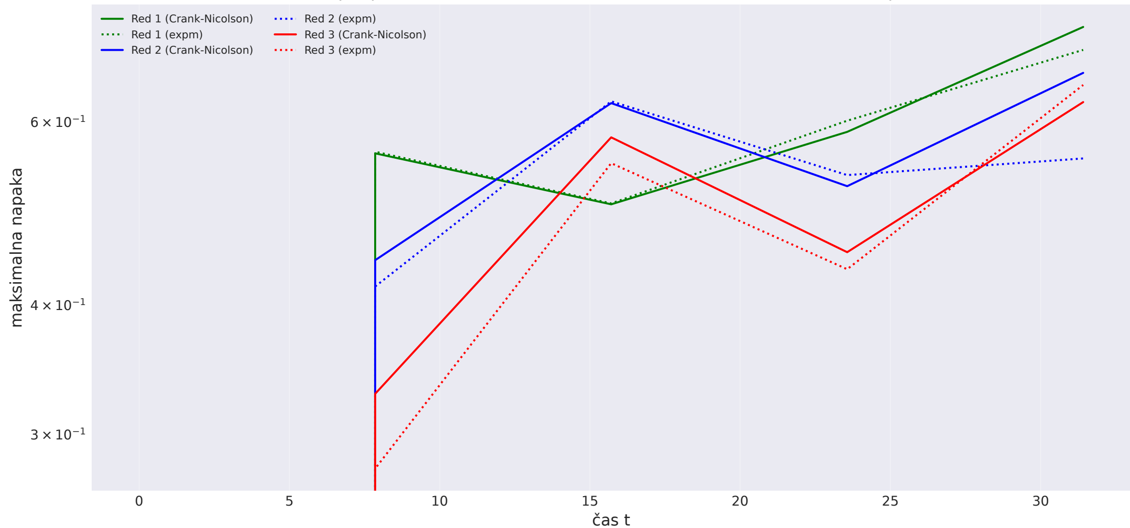
Največja absolutna vrednost razlike med numerično in analitično rešitvijo
