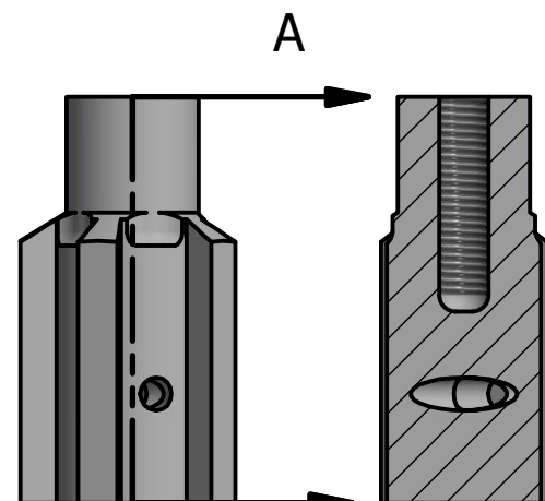
A QUERSCHNITT A-A MASSSTAB 2 : 1
