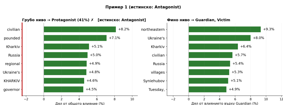
Фигура 5.1: Дял на влиянието на водещите думи за Случай 1 (обект Russia ): грешна класификация Antagonist → Protagonist.
