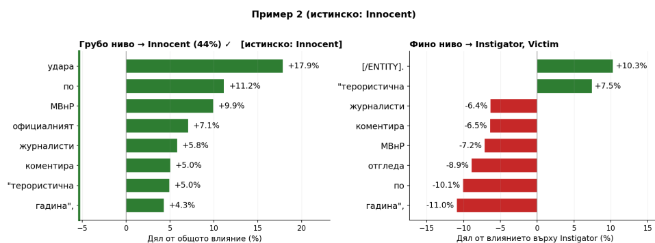
Фигура 5.2: Дял на влиянието на водещите думи за Случай 2 (обект Луганск ): правилна класификация Innocent.
