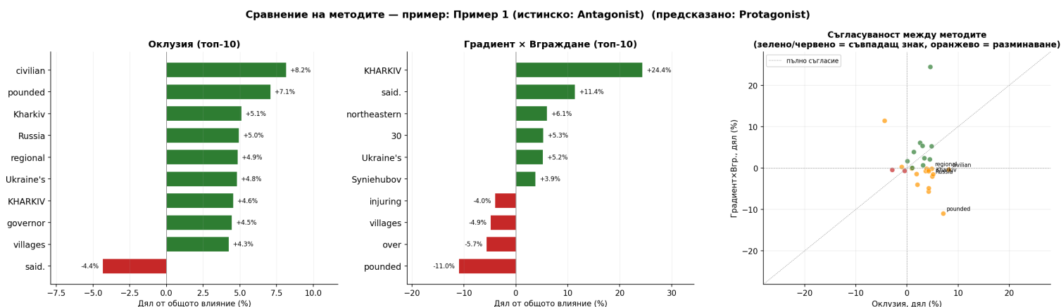
Фигура 5.3: Сравнение на оклузионен анализ и градиент × вграждане за примера с Russia .
