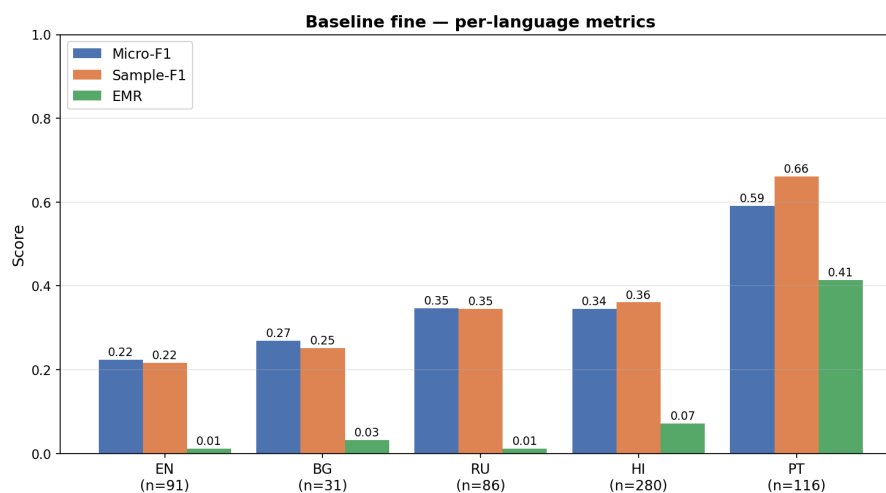
Фигура 4.6: Sample-F1 на финия класификатор по езици.
