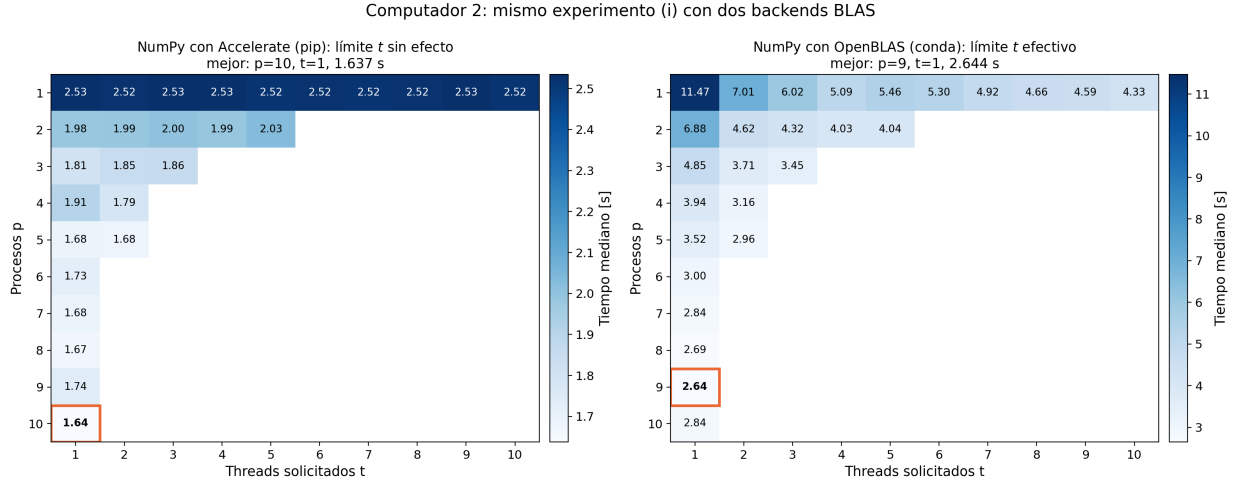
Figura 5: Inciso (i) en el computador 2: experimento original (izquierda) y repetición con el límite de threads efectivo (derecha).
