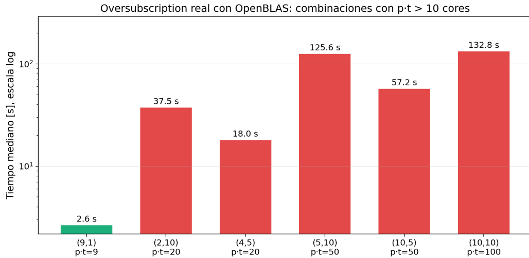
Figura 6: Oversubscription provocada en el computador 2 con combinaciones pt > 10 . Eje vertical en escala logarítmica.
