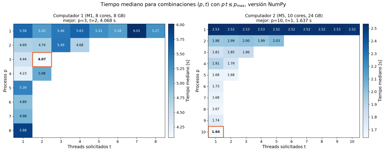
Figura 8: Tiempo mediano de la versión NumPy para cada combinación (p, t) con p \leq p_{\max} . La celda destacada es la mejor de cada computador.
