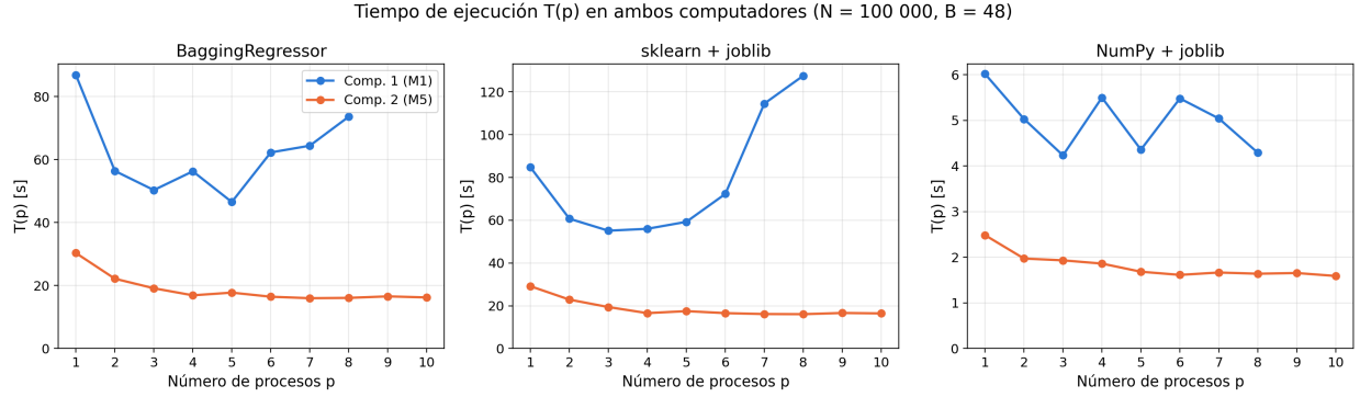
Figura 5: Tiempo mediano T(p) en ambos computadores, un panel por implementación. El computador 1 llega hasta p = 8 y el computador 2 hasta p = 10 .
