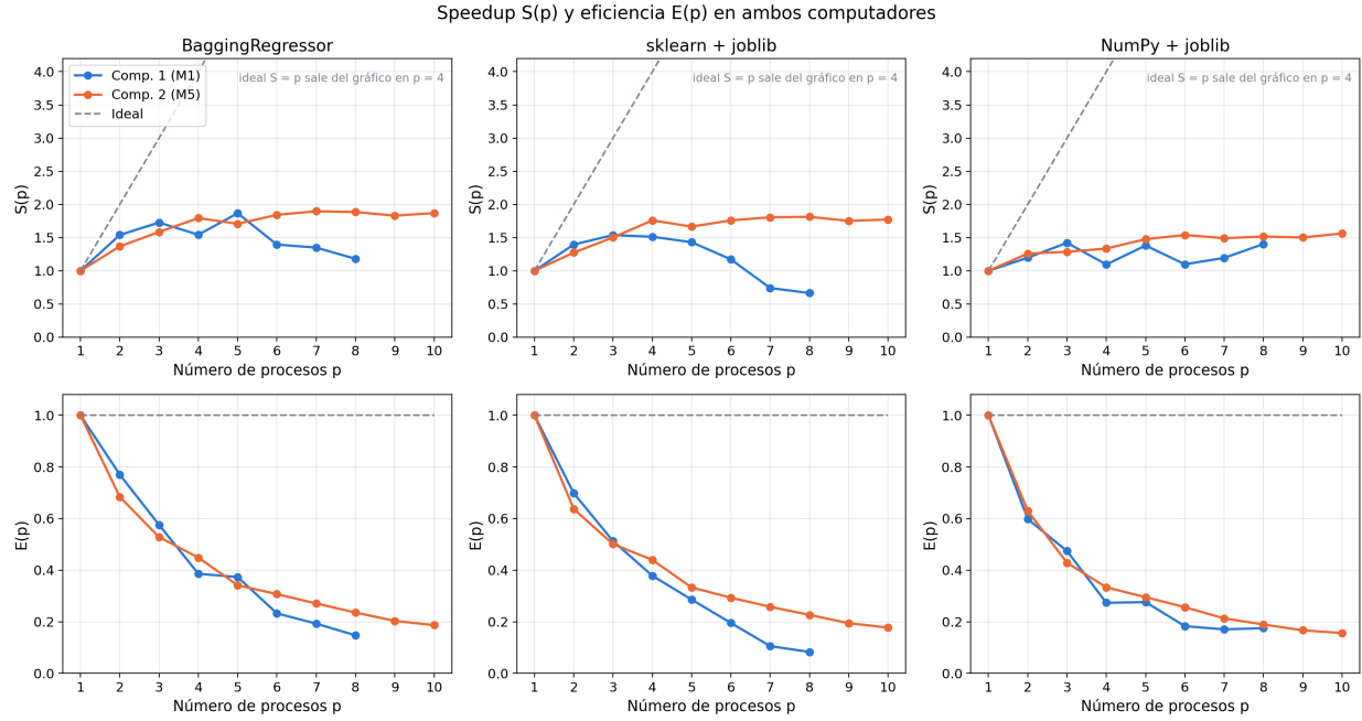
Figura 6: Speedup S(p) (arriba) y eficiencia E(p) (abajo) en ambos computadores. La línea discontinua es la curva ideal.
