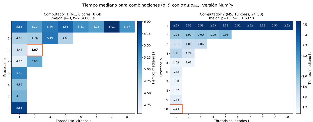
Figura 8: Tiempo mediano de la versión NumPy para cada combinación; en naranja, el más rápido.
