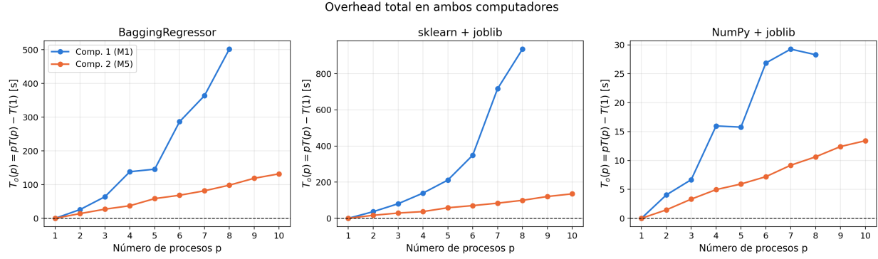
Figura 7: Overhead total T_o(p) = pT(p) - T(1) en ambos computadores.
