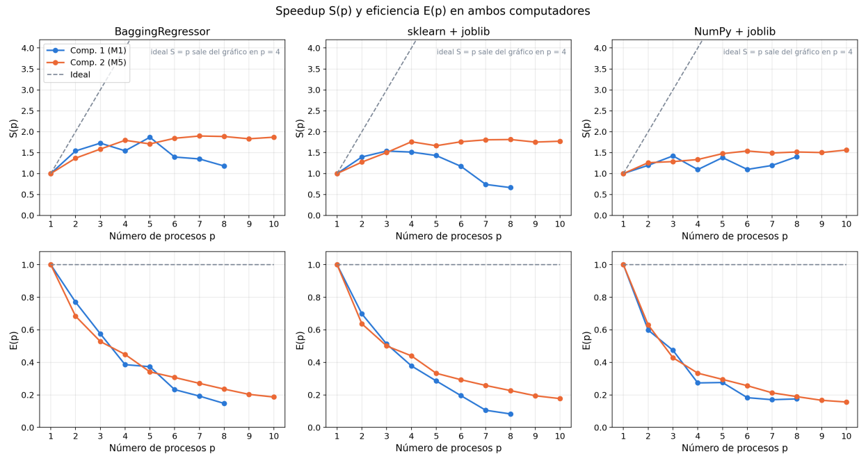
Figura 7: Speedup S(p) (arriba) y eficiencia E(p) (abajo) en ambos computadores.
