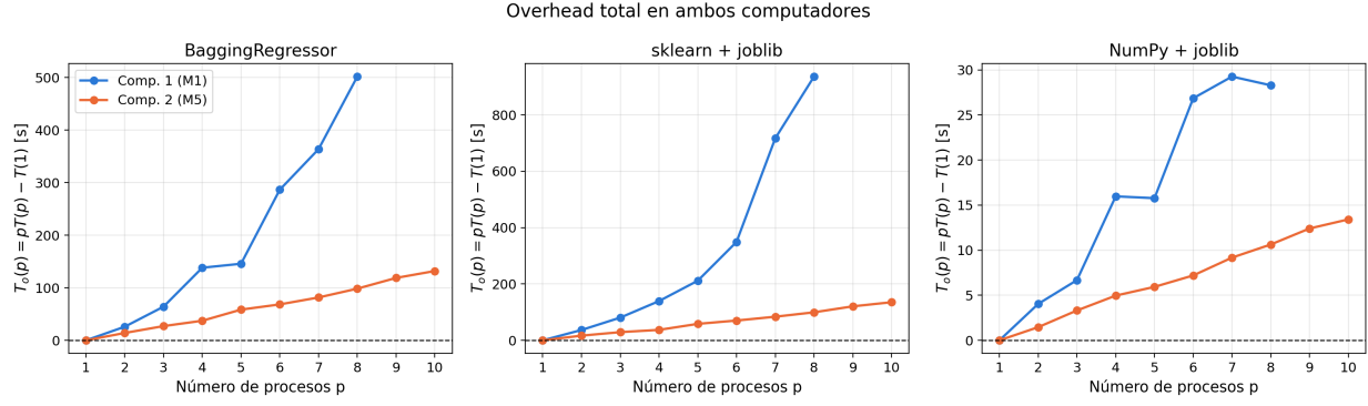
Figura 8: Overhead total T_o(p) = pT(p) - T(1) en ambos computadores.
