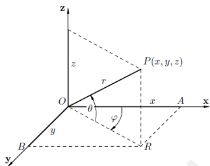
Rysunek 2: Sferyczne współrzędne.
