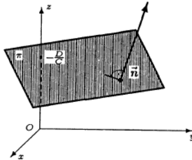
Rysunek 6: Płaszczyzna i wektor normalny.
