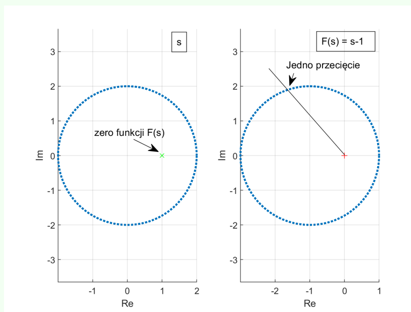
Rysunek 3: Zasada argumentu dla funkcji F(s) = s - 1 i konturu zdefiniowanego jako okrąg o promieniu 2 i środkiem w punkcie (0,0) .
