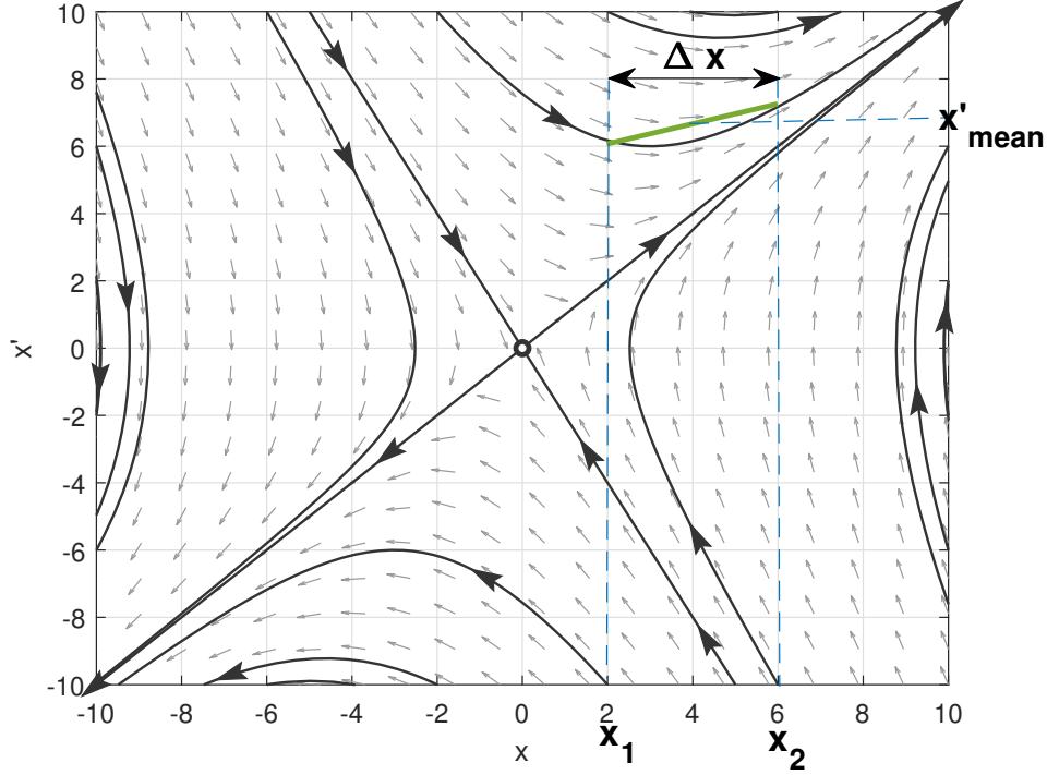
Rysunek 2: Aproksymacja trajektorii fazowej odcinkami.
