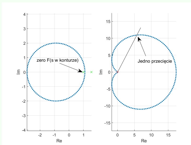
Rysunek 5: Zasada argumentu dla funkcji F(s) = (s - 1)(s - 1.55) i konturu zdefiniowanego jako okrąg o promieniu 2 i środkiem w punkcie (-0.9,0).
