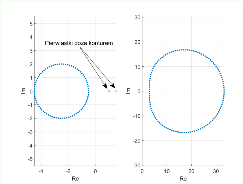
Rysunek 6: Zasada argumentu dla funkcji F(s) = (s - 1)(s - 1.55) i konturu zdefiniowanego jako okrąg o promieniu 2 i środku w punkcie (-2.5, 0) .
