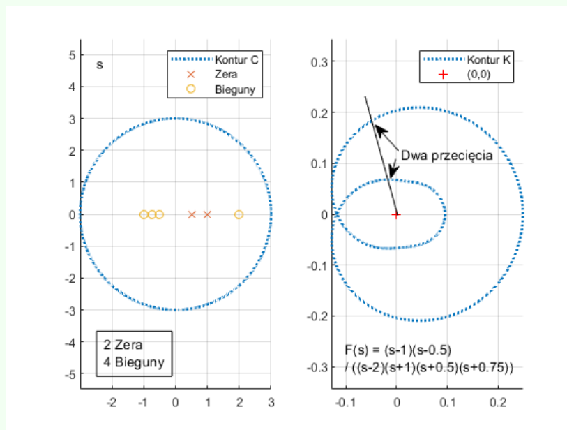
Rysunek 7: Zasada argumentu dla funkcji F(s) = \frac{(s-1)(s-0.5)}{(s-2)(s+0.5)(s+1)(s+0.75)} i konturu zdefiniowanego jako okrąg o promieniu 3 i środku w punkcie (0, 0) .
