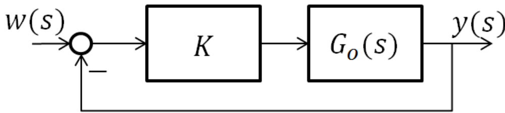
Rysunek 1: Zamknięty układ regulacji.
